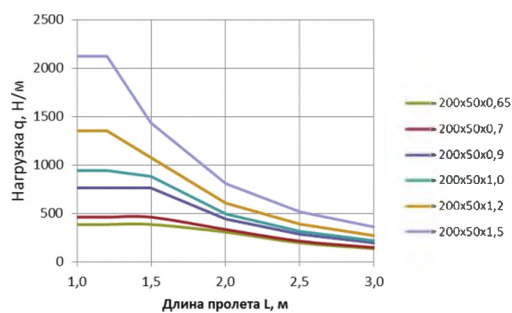
БРН для лотков 200х50
