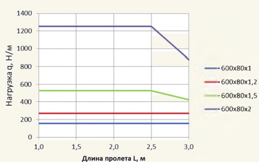
БРН для лотков 600x80
