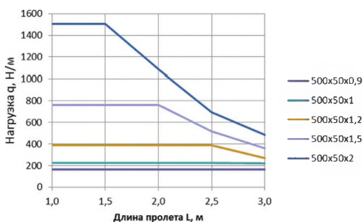
БРН для лотков 500х50
