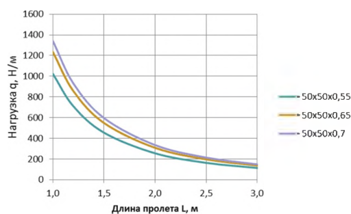
БРН для лотков 50х50
