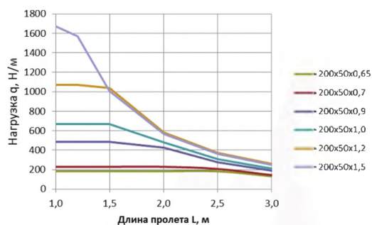
БРН для лотков ЛП 200х50
