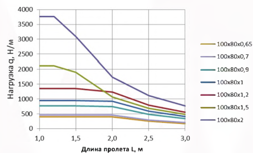
БРН для лотков ЛП 100х80
