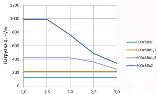
БРН для лотков ЛП 600х50
