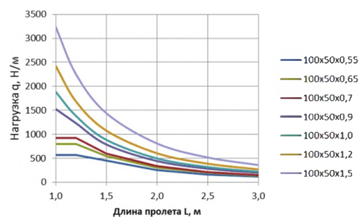
БРН для лотков 100х50
