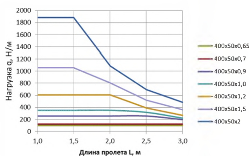
БРН для лотков 400х50
