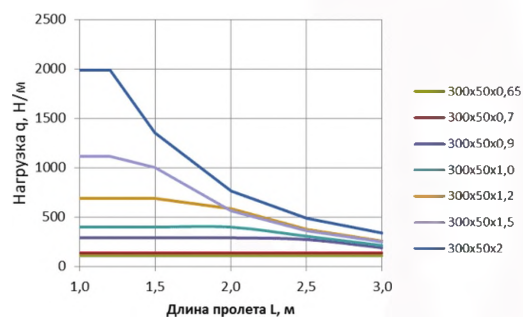
БРН для лотков ЛП 300х50
