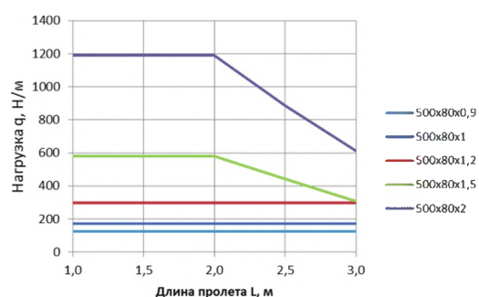
БРН для лотков ЛП 500x80
