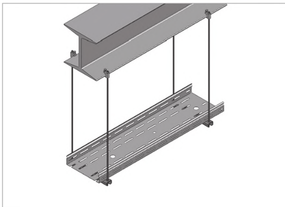
Крепление лотка к строительным конструкциям Крепление лотка к двутавру с помощью сборного подвеса (4 струбины + 4 шпильки + 2 профиля монтажных)
