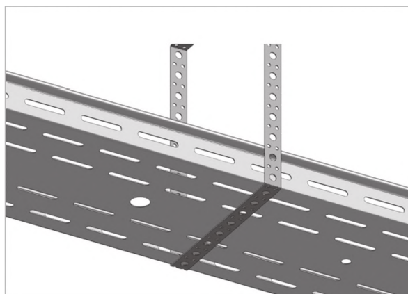
Крепление лотка к потолку с помощью перфоленты
