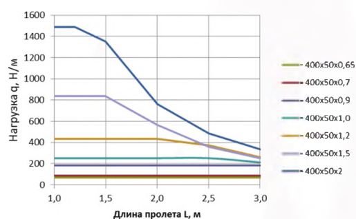
БРН для лотков ЛП 400х50
