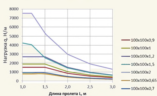
БРН для лотков 100x100
