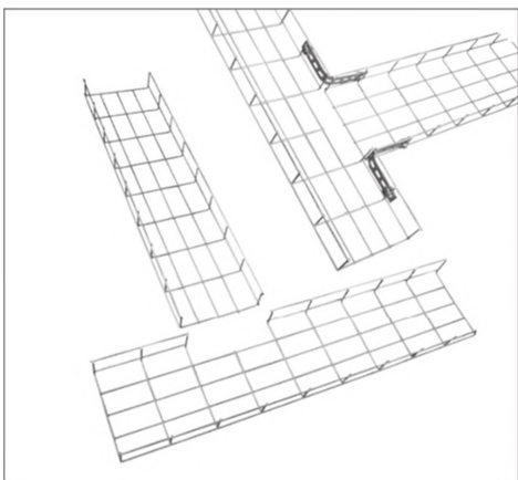
Ответвитель Т-образный
