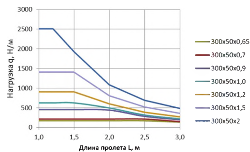
БРН для лотков 300х50
