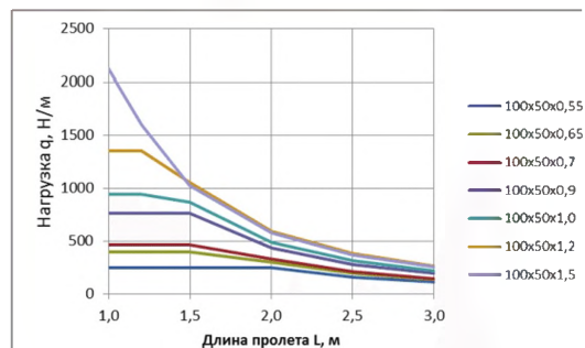
БРН для лотков ЛП 100х50
