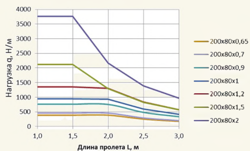
БРН для лотков 200x80
