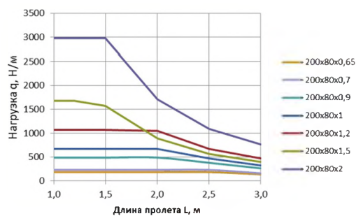
БРН для лотков ЛП 200x80
