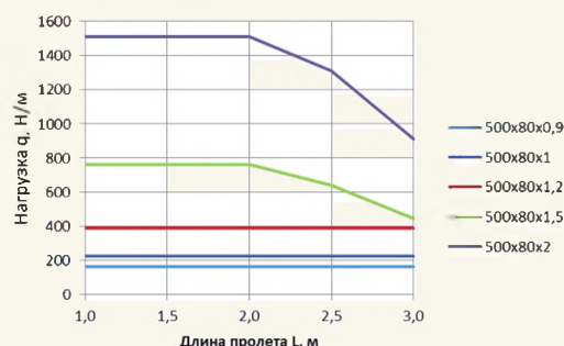
БРН для лотков 500x80
