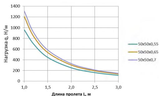
БРН для лотков ЛП 50х50
