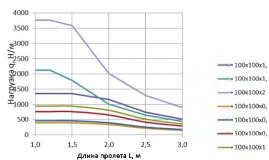
БРН для лотков ЛП 100x100
