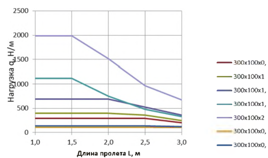
БРН для лотков ЛП 300x100
