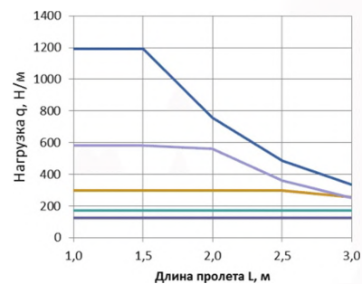
БРН для лотков ЛП 500х50
