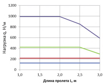
БРН для лотков ЛП 600x80
