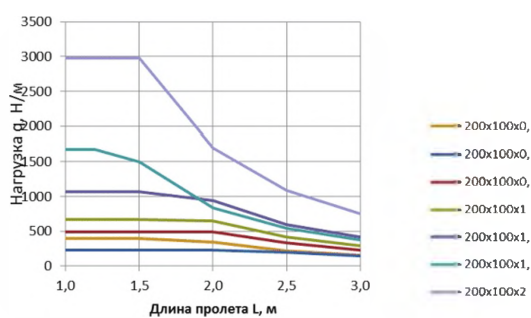
БРН для лотков ЛП 200x100
